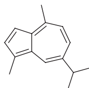
11. Guaiazulene
