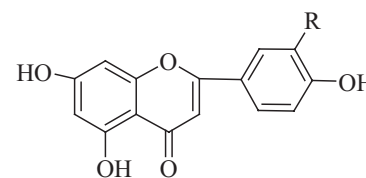
16. Apigenin (R=H)
