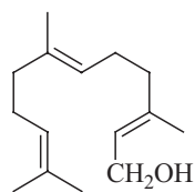
5. Farnesol
