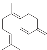
4. \beta -Farnesene
