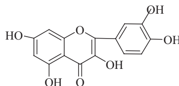
20. Quercetin
