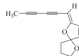
21. Z-Enyne dicycloether
